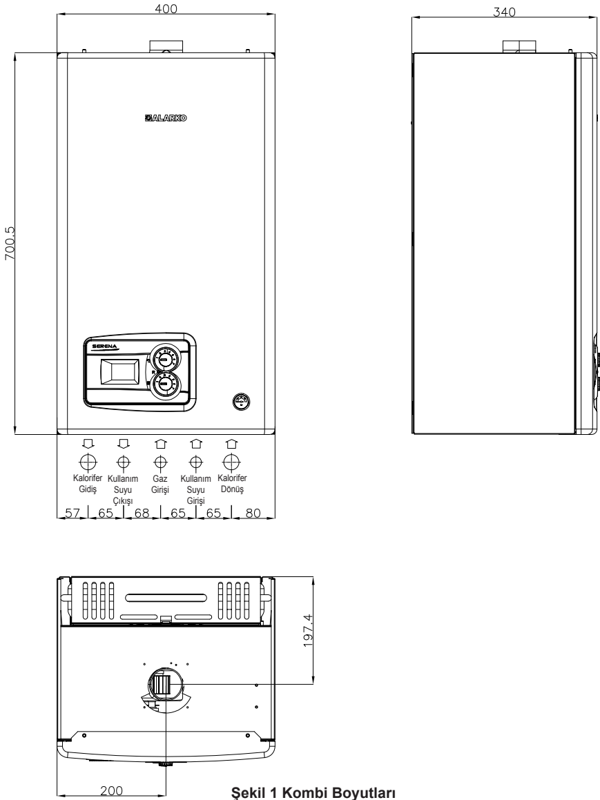
Şekil 1 Kombi Boyutları
