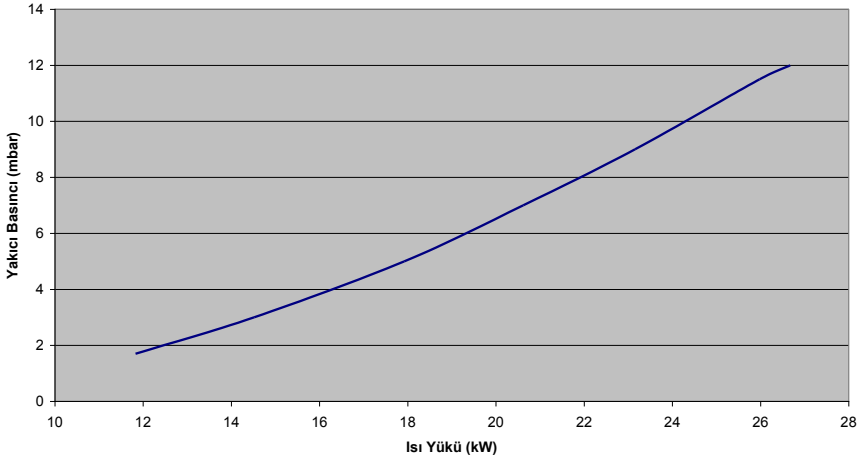
Şekil 25 Yakıcı Basıncı - Isıtma Yükü Diagramı
