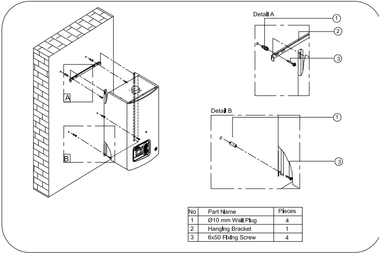
Şekil 11 Duvara Montaj Şeması
