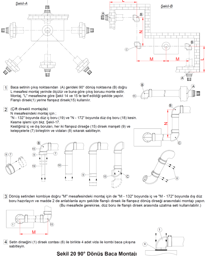
Şekil 20 90° Dönüş Baca Montajı
