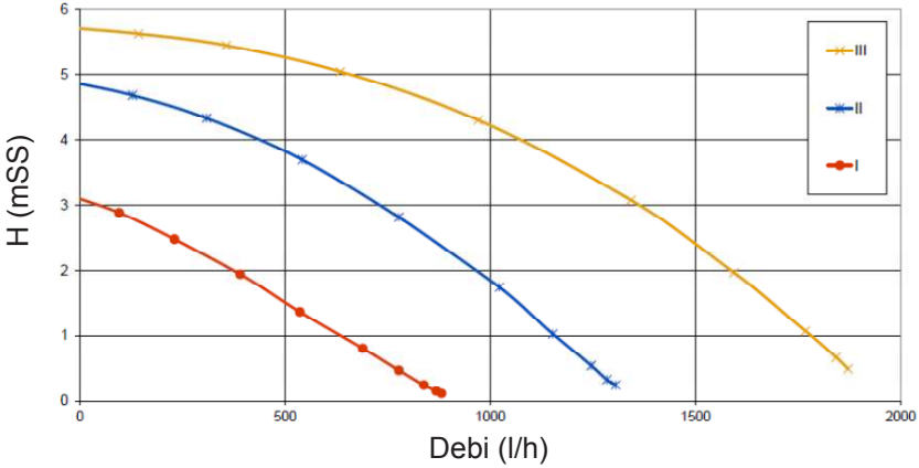
Şekil 23 Sirkülasyon Pompası Performans Grafiği
