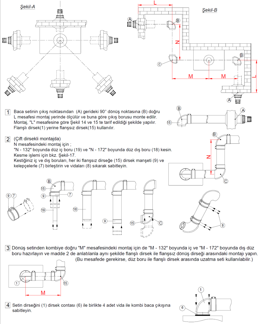
Şekil 17 Standart Baca Seti Montajı
