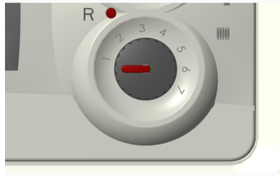
Şekil 6 Kalorifer Sistemi Ayar Düğmesi
